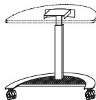
8G Gasdrivet stativ 800×400 mm höjd 728–1128 mm (exkl. skiva)
